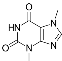
Teobromin
